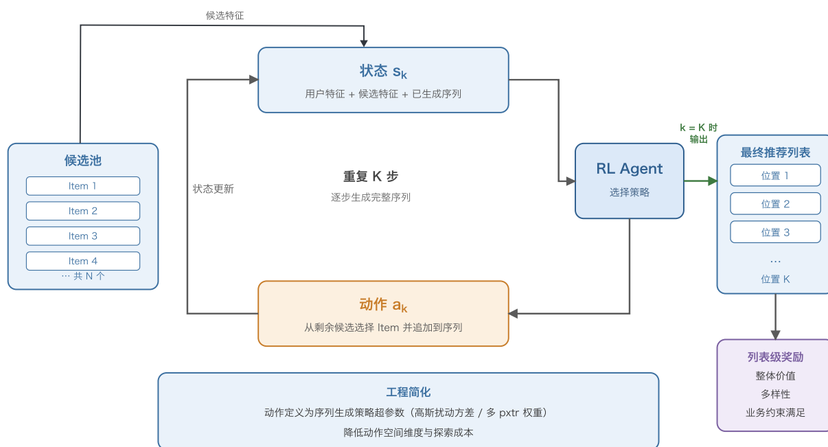
图 28.6: 强化学习序列生成的逐步决策过程。
